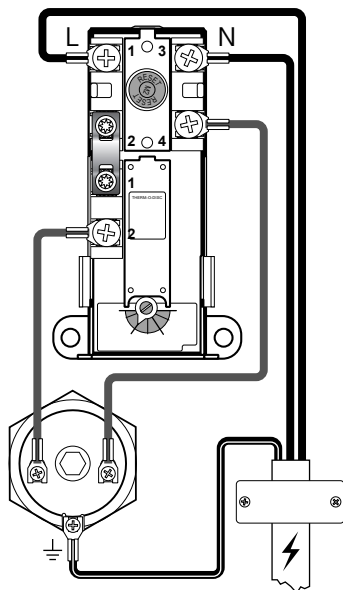
Połączenie elektryczne, schemat
