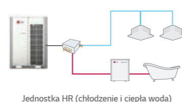
Jednostka HR (chłodzenie i ciepła woda)
