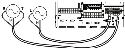
Grzałka rezerwowa 3Ø (Dla Hydrosplit)
