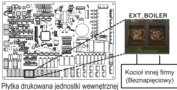
Płytką drukowaną jednostki wewnętrznej
