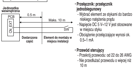
Przykładowa instalacja #1
