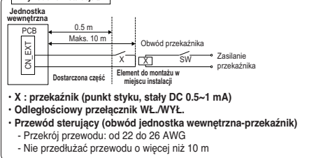
Przykładowa instalacja #2
