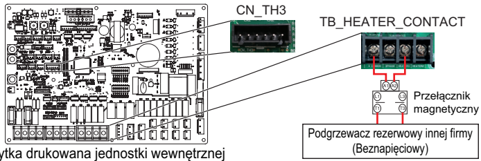
Płytką drukowaną jednostki wewnętrznej
