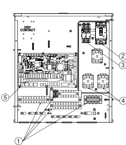
Z przełącznikiem magnetycznym (Data produkcji : Do 30 września 2019)
