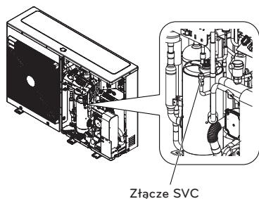
Złącze SVC
