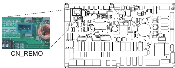
Płytką drukowaną jednostki wewnętrznej
