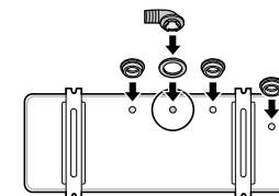
Króciec spustowy
