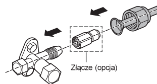
Króciec spustowy
