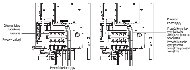
Główna listwa zaciskowa zasilania
