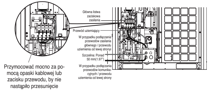
Połączenie przewodu komunikacyjnego/uziemienia
