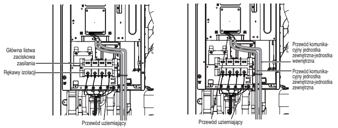
Podłączenie linii zasilania głównego
