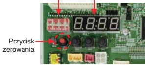
Przełącznik DIP 7 - segmentowy
