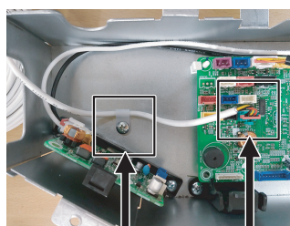
Zacisk przewodu
