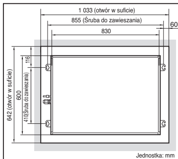
Podstawa TS
