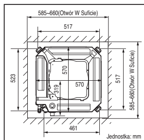
Podstawa TQ/TR
