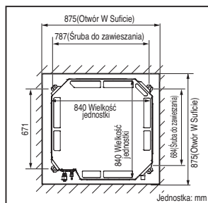
Podstawa TM/TN/TP/TM-A/TP-B
