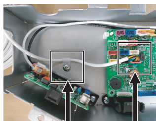
Złącze kontrolera przewodowego (CN-REMO)
