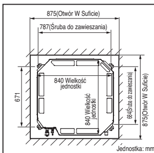
Podstawa TM/TN/TP/TM-A/TP-B
