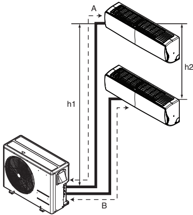
Multisplit
