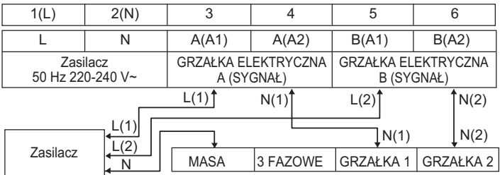
(1Ø 6 kW) Blok przyłączeniowy 2 (W grzałce elektrycznej)
