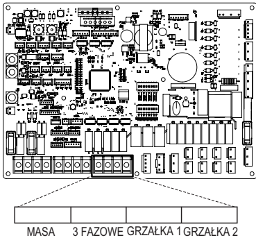
Płyta drukowana jednostki wewnętrznej
