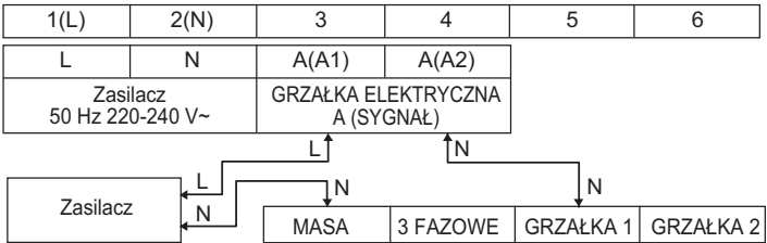
(1Ø 3 kW) Blok przyłączeniowy 2 (W grzałce elektrycznej)
