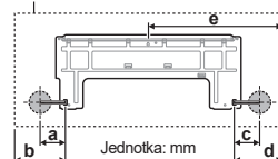
Rám vnitřní jednotky
